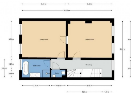
Nieuwe Schoolstraat 2A, Den Haag | 1e Verdieping H = 3.68 m
