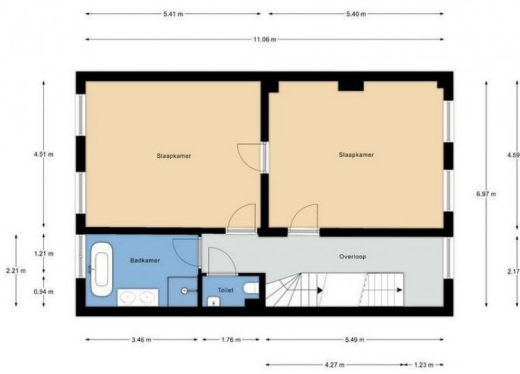
Nieuwe Schoolstraat 2A, Den Haag | 1e Verloping H = 3,68 m
