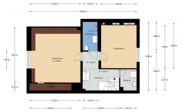
Nieuwe Schoolstraat 2A, Den Haag | 2e Verloping H = 2,22 - 4,06 m
