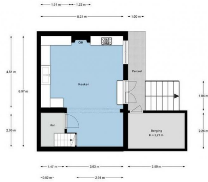
Nieuwe Schoolstraat 2A, Den Haag | Souterrain H = 2,24 m
