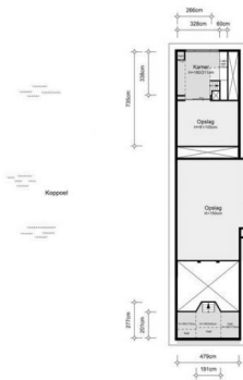
POELDIJK 1B te RIJPWETERING WOONBOOT LAGE DEEL
